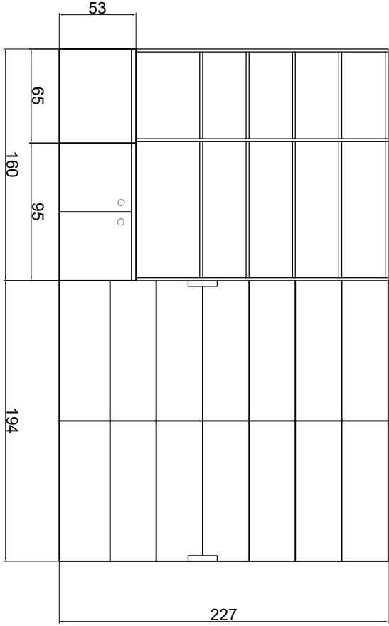
SEZ. B-B
